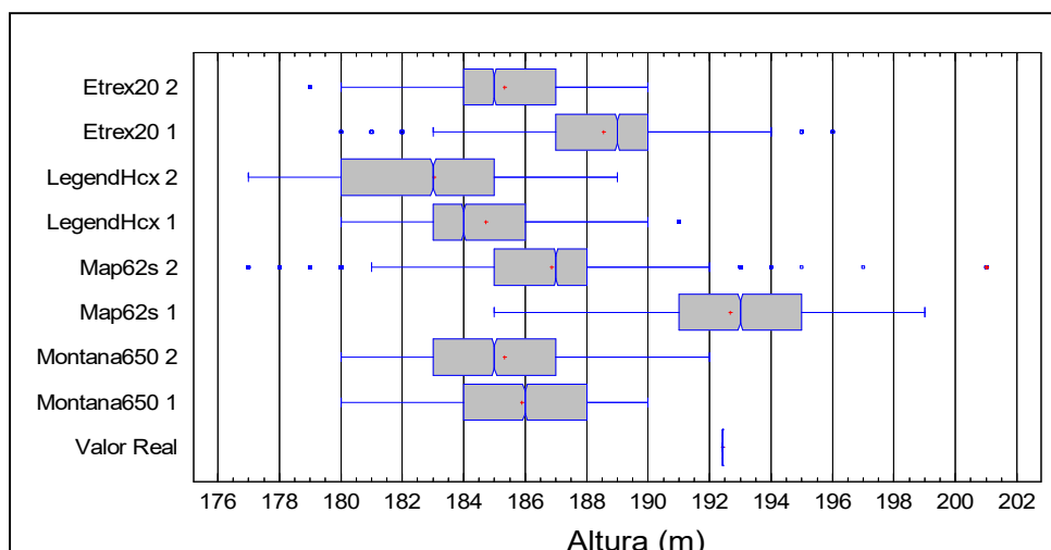
Gráfico 3: Comportamiento de los registros de altitud de los cuatro navegadores en los dos días, con respecto al valor verdadero. (Los números 1 y 2 se refieren a los días). Graph 3: Behavior of altitude records for the four navigators in the two days, with respect to the true value. (Numbers 1 and 2 refer to days).
