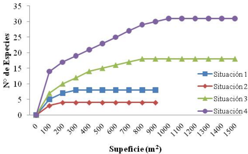
Gráfico 1: Curvas de acumulación de especies en el estrato arbóreo. Graph 1: Curves of accumulation of species in the tree stratum.
