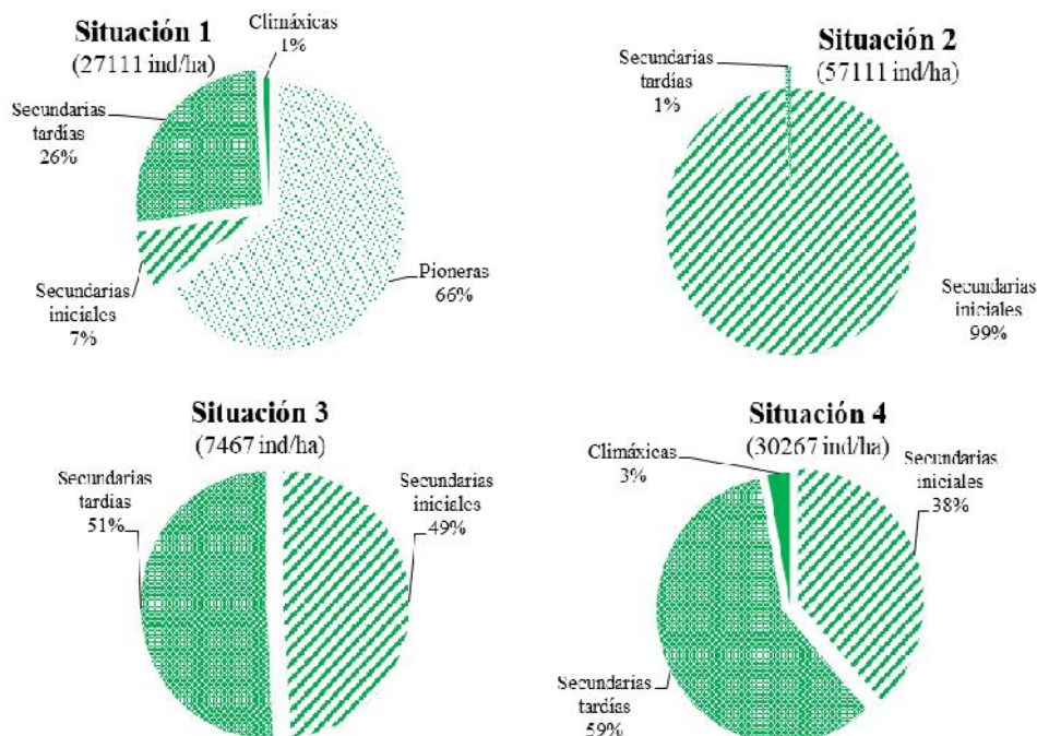
Gráfico 6: Proporción de individuos por grupo ecológico para las situaciones. Graph 6: Proportion of individuals by ecological group for each situations.
