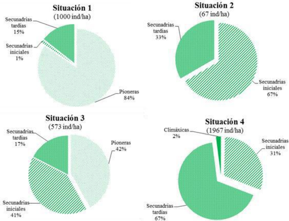
Gráfico 3: Proporción de individuos arbóreos por grupo ecológico para las situaciones. Graph 3: Proportion of arboreal individuals per ecological group for situations.
